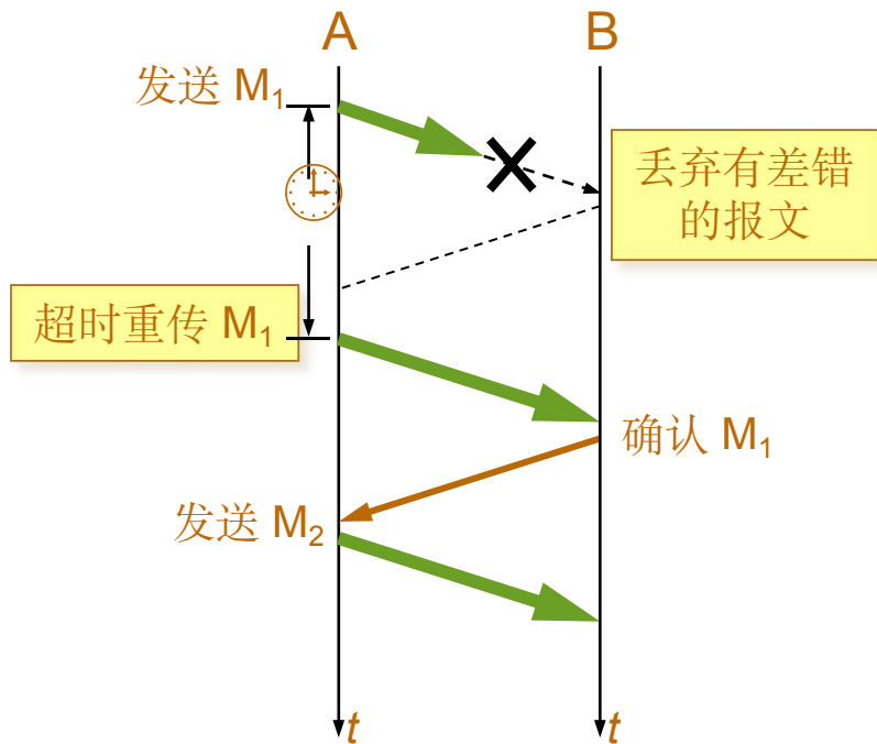
(b) 超时重传
